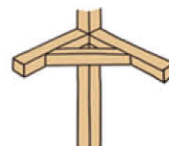
火打ち梁
