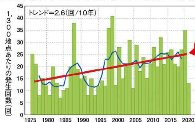
全国の1時間降水量80ミリ以上の年間発生回数の経年変化
